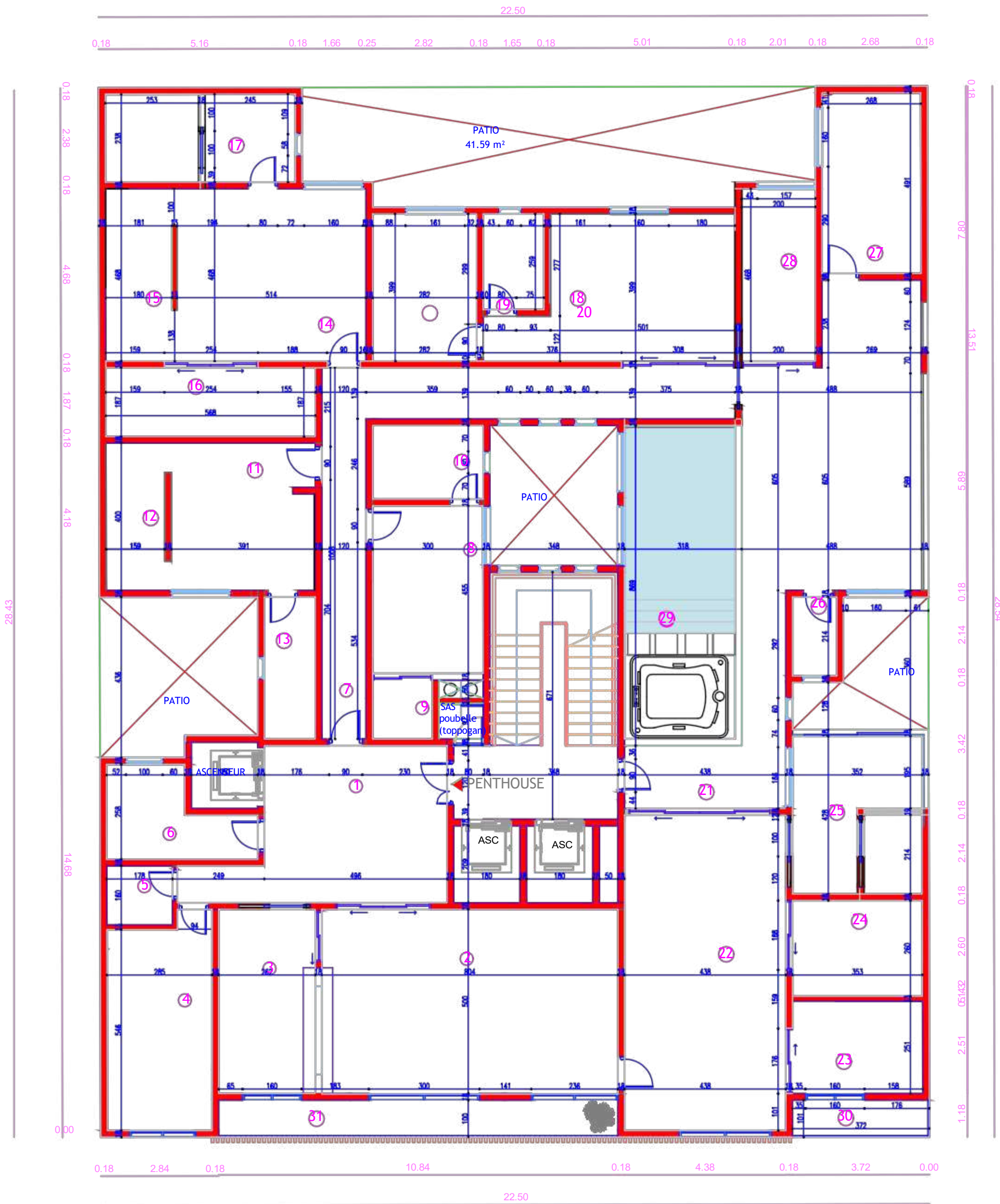
Plan MAÇONNERIE
