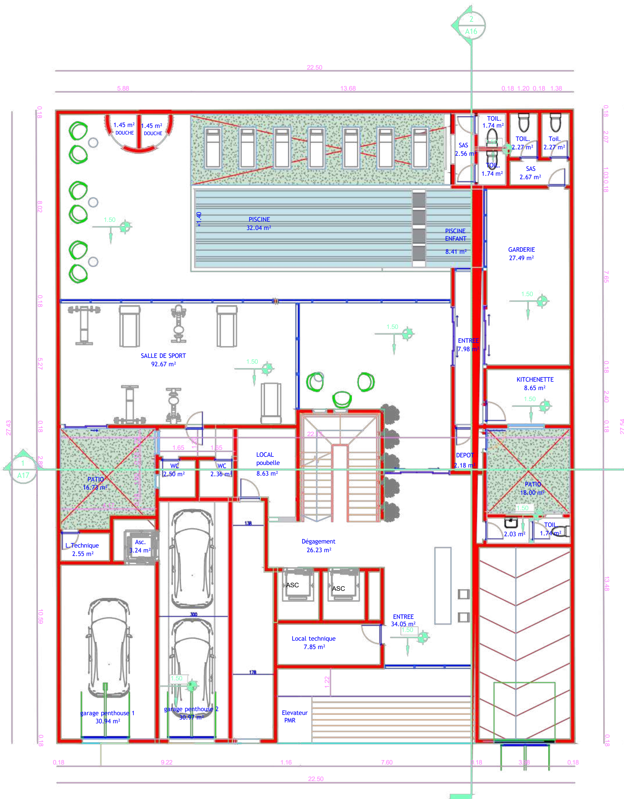
Plan D'AMENAGEMENT
