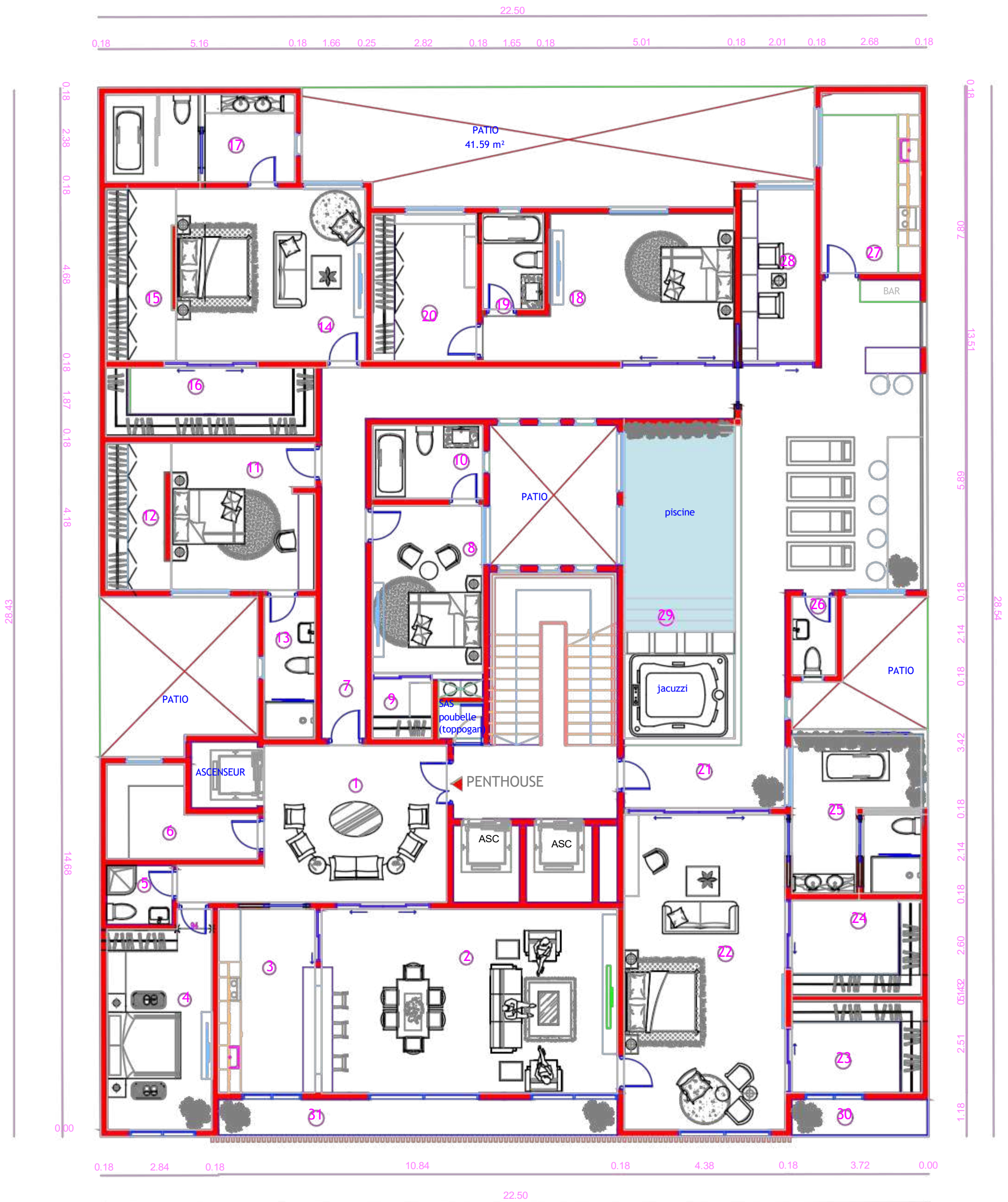
Plan D'AMENAGEMENT
