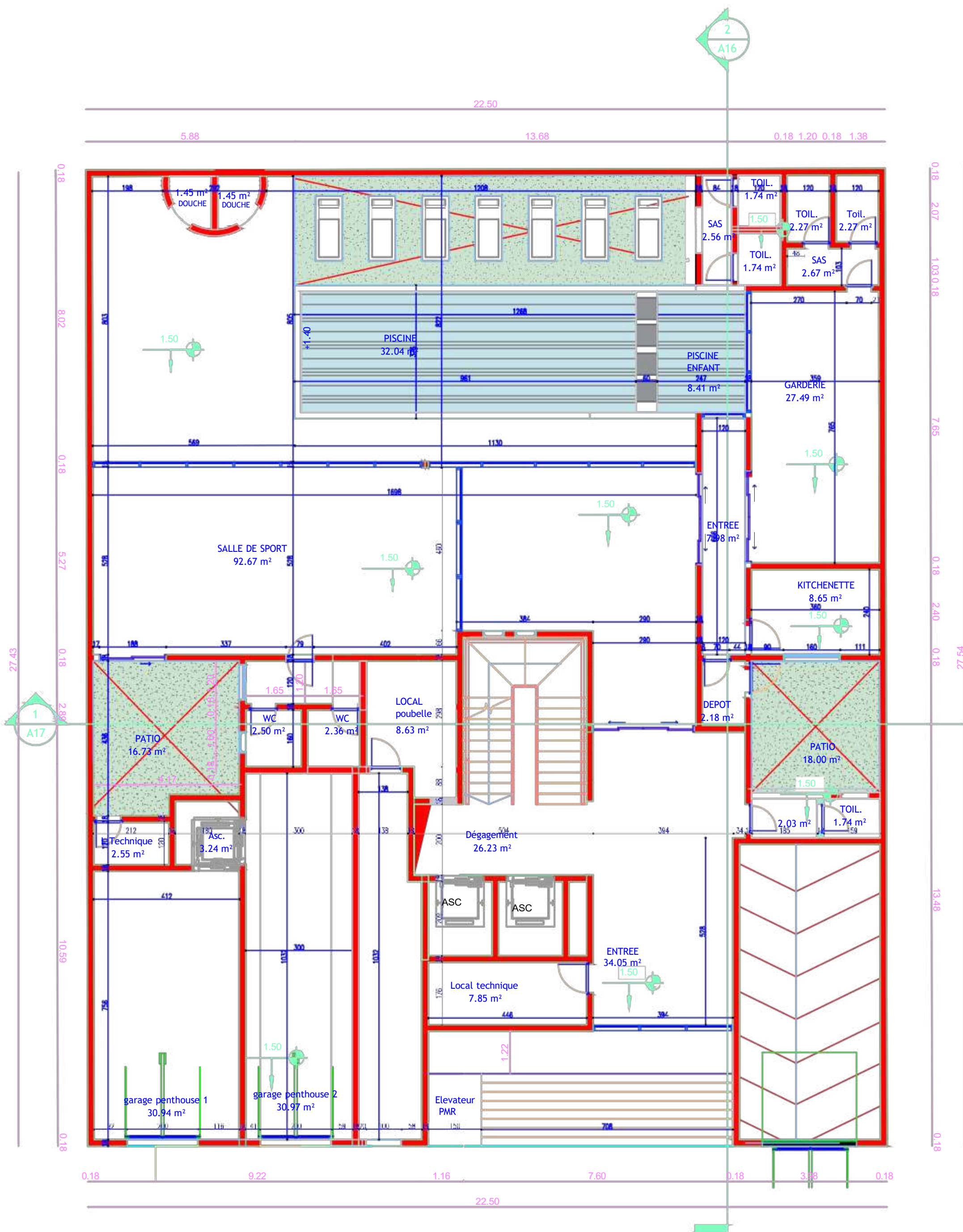
Plan MAÇONNERIE
